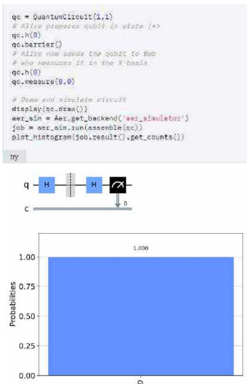
Рис. 10. Выходные данные и результаты работы алгоритма
