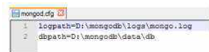
Рисунок 4.2 Содержание файла конфигурации MongoDB.
