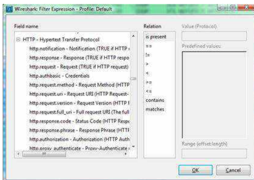
Рис. 1.5. Свойства HTTP-пакета для использования в фильтре
