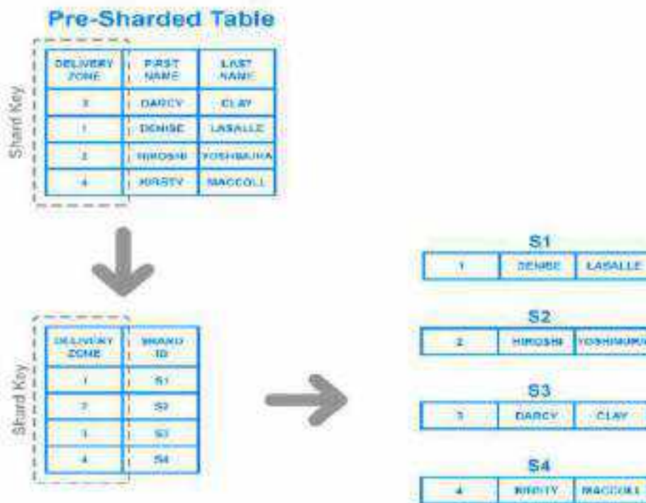
Рисунок 2.4 – Упрощенный пример шардинга на основе каталога
