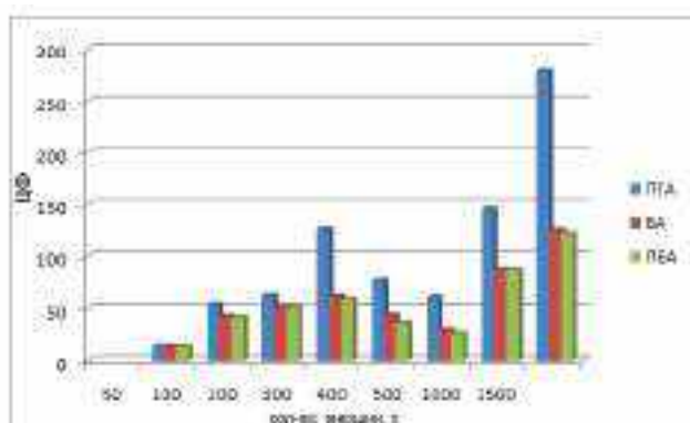
Рис. 5. Гистограмма зависимости изменения ЦФ от количества вершин графа для задачи о кратчайшем пути
