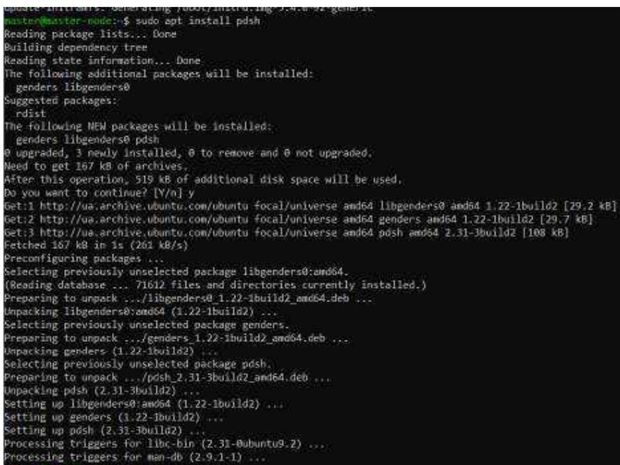
Рис. 10 — процесс установки pdsh
