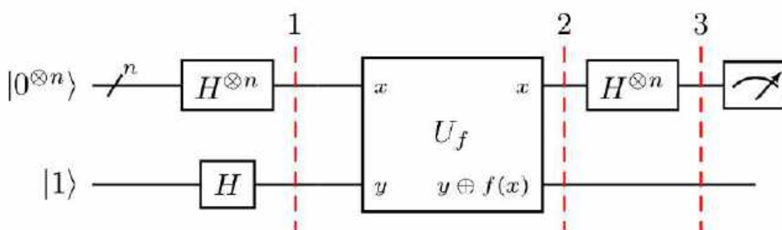
Рис. 14. Общая схема алгоритма Дойча-Джозса
