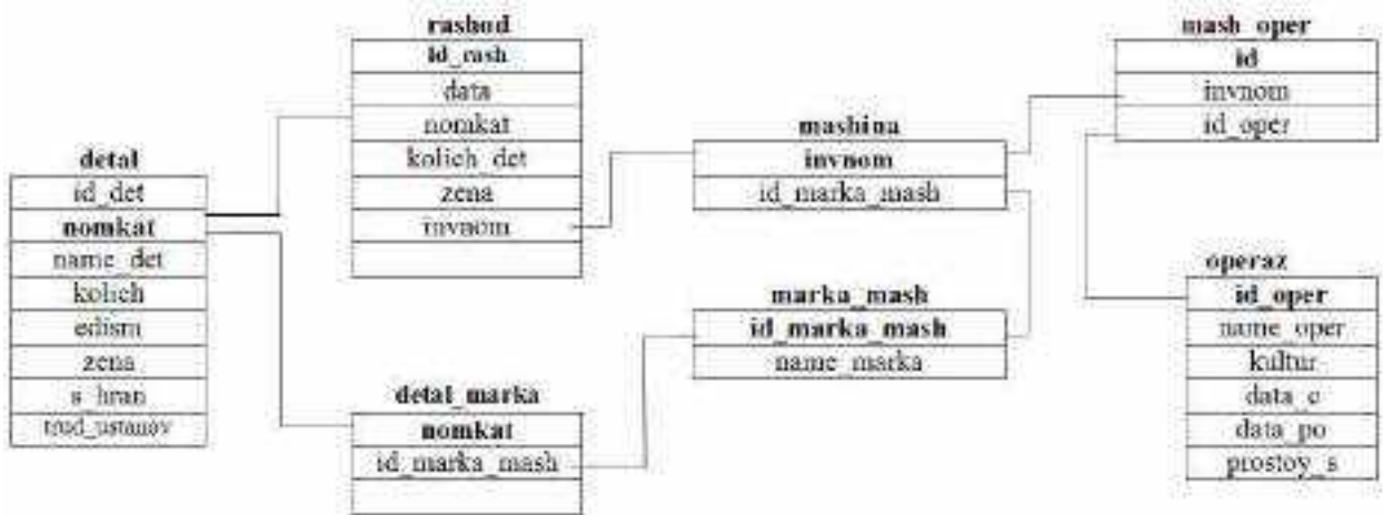
Рисунок 1.1. – ER- диаграмма модели данных информационной системы для резервирования запасных частей сельскохозяйственной техники
