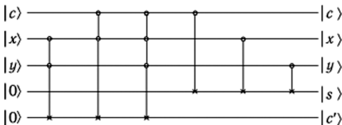
Рис. 5.43. Графическое изображение квантового сумматора
