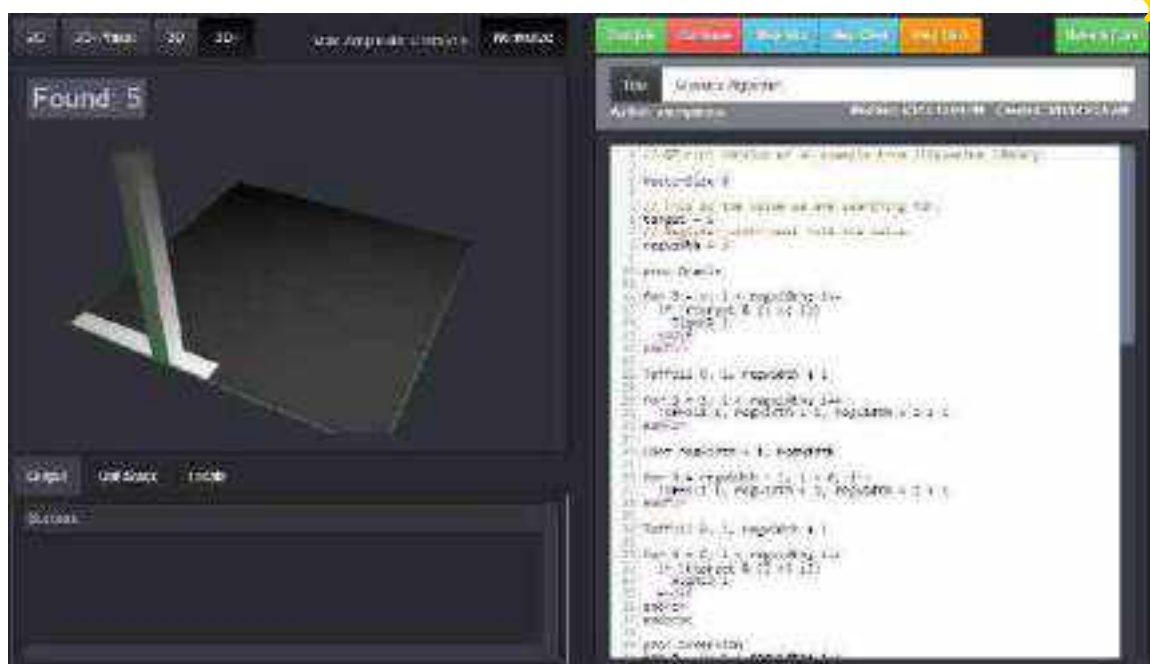
Рис. 13. Реализация квантового поискового алгоритма Гровера от Google
