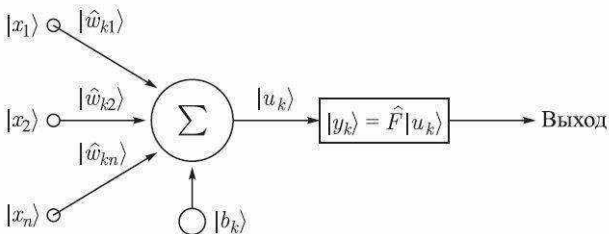
Рис. 5.41. Блок-схема квантового нейрона
