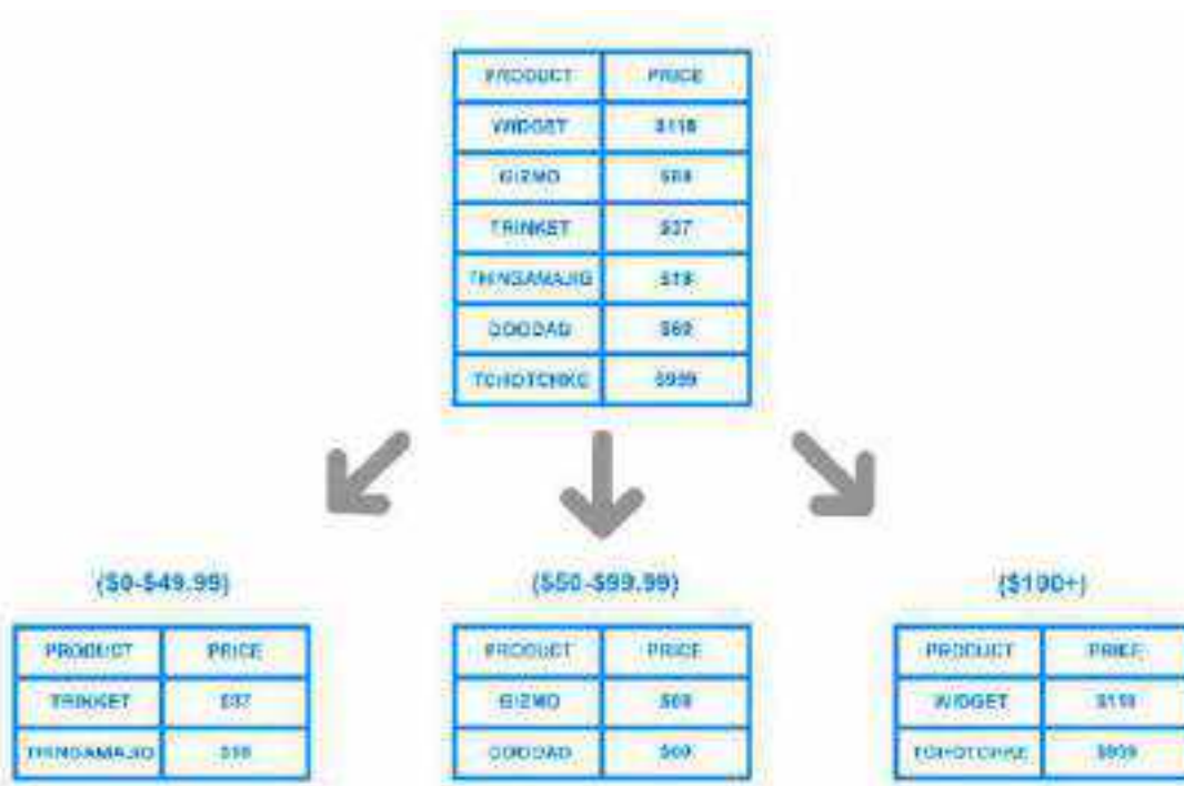
Рисунок 2.3 – Шардинг на основе диапазона
