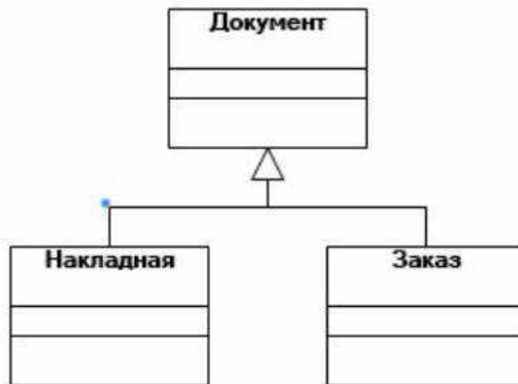
Рисунок 5 – Наследование
