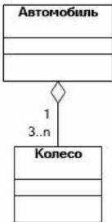
Рисунок 3 – Агрегация
