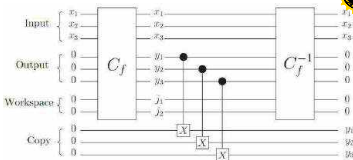
Рис. 4. Схема для обратимого вычисления f(x)
