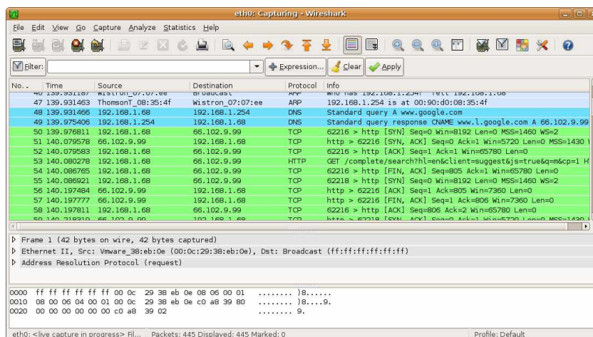
Рис. 1.4. Пакеты в Wireshark без фильтра
