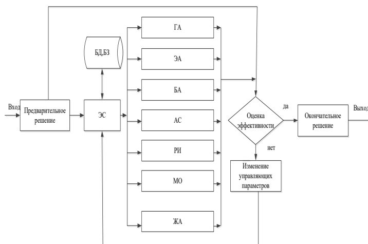
Рис. 1. Упрощенная схема интегрированного поиска
