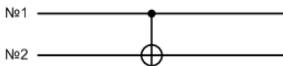
Рис. 5.42. Графическое изображение гейта CNOT
