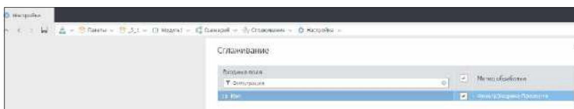
Рисунок 6.5 Выбор метода сглаживания данных
