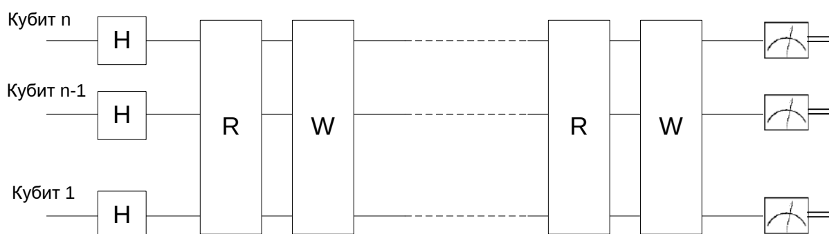
Рис. 12. Квантовая сеть алгоритма Гровера
