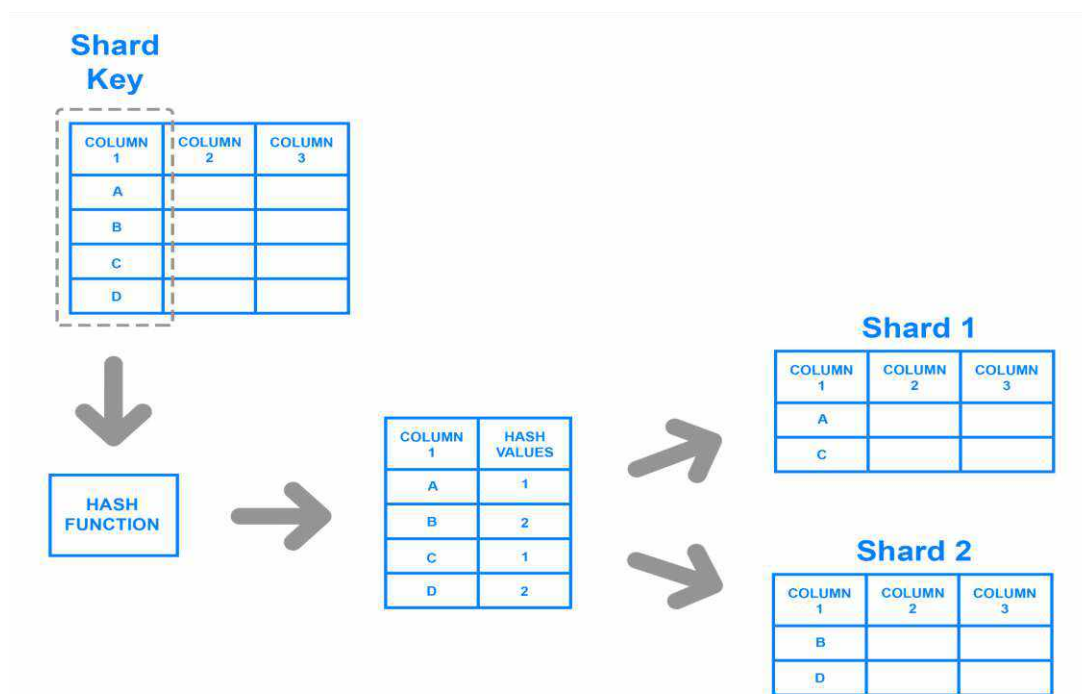
Рисунок 2.2 – Шардинг на основе ключей
