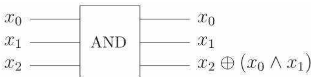
Рис. 3. Реверсивный вентиль AND
