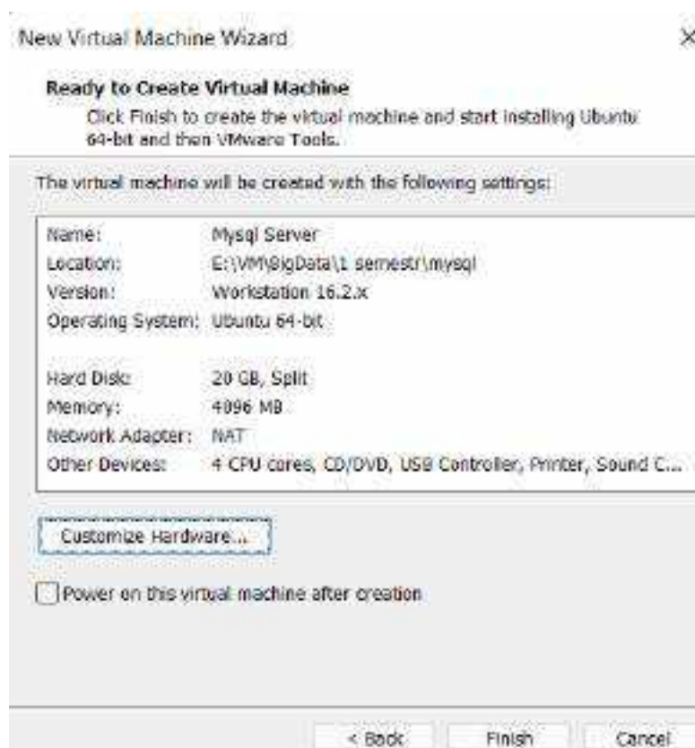
Рис.1 — Характеристики виртуальной машины
