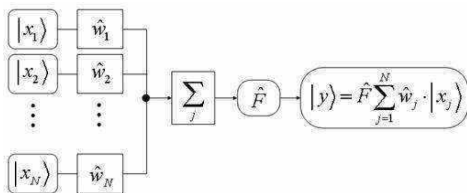
Рис. 5.21. Математическая модель нейрона
