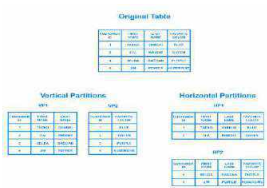
Рисунок 2.1 – Вертикальное и горизонтальное разделение таблицы
