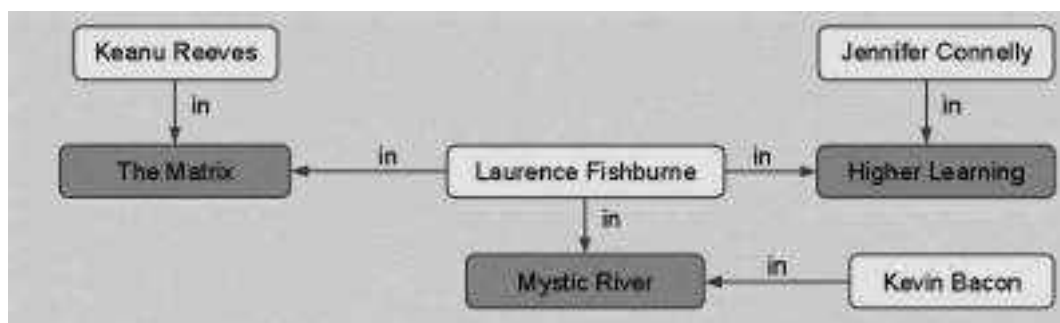
Рисунок 5.2 Фрагмент модели данных
