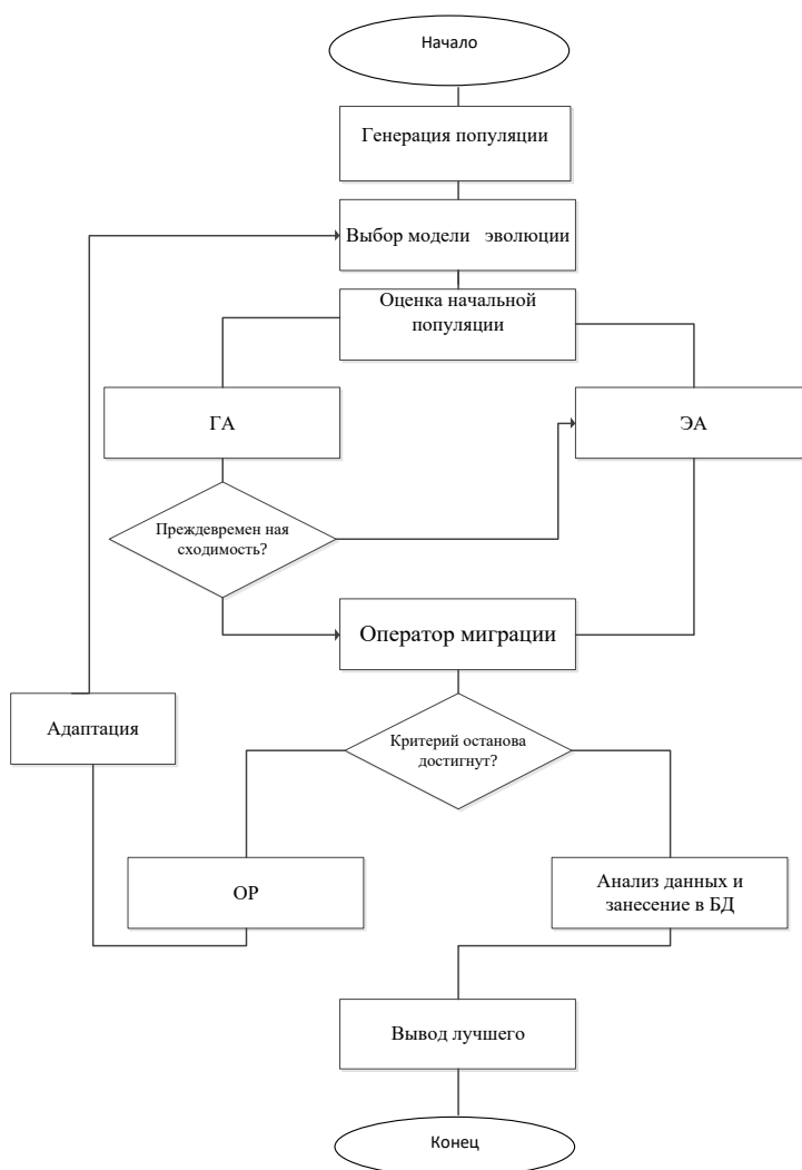
Рис. 2 Обобщенная схема биоинспирированного поиска для задачи об экстремальном пути
