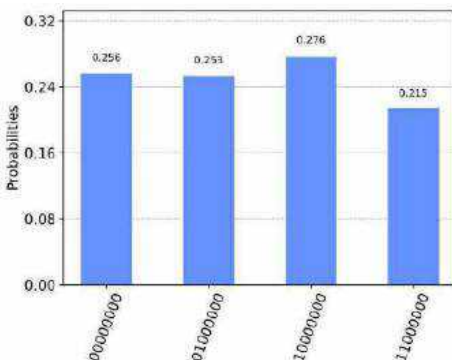
Рис. 9. Выходные данные и результаты работы алгоритма
