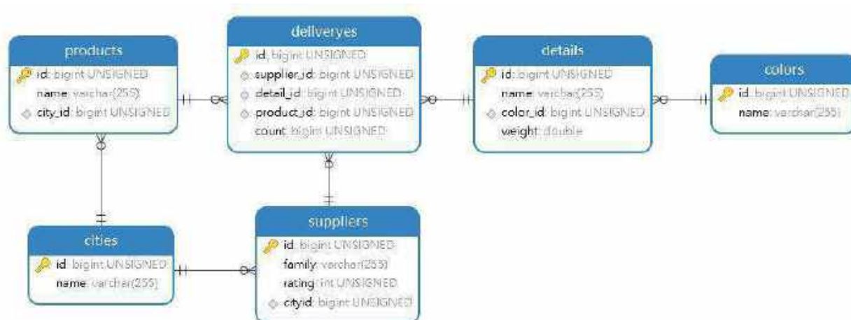
Рис. 17 — Разработанная структура базы данных
