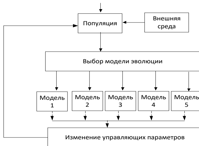
Рис. 3. Условная упрощенная интегрированная схема эволюции
