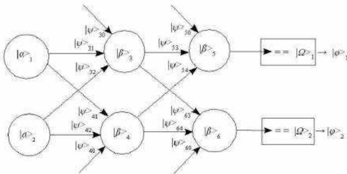
Рис. 5.44. КНС, вычисляющая XOR-функции
