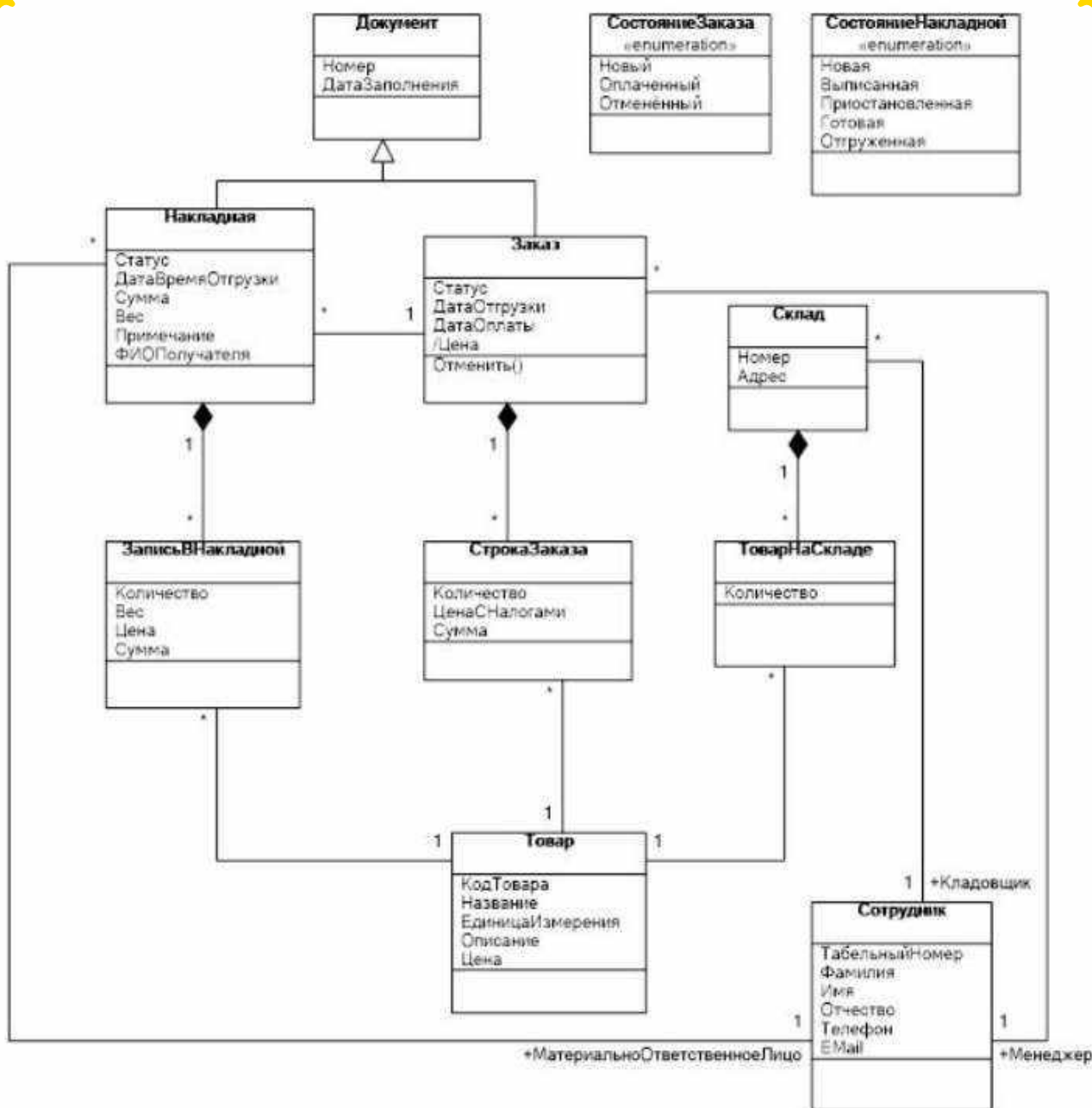
Рисунок 6 – Диаграмма классов
