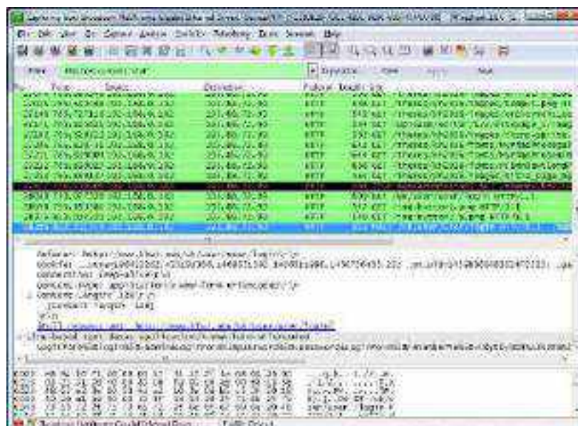
Рис. 1.7. Пакет с логином и паролем
