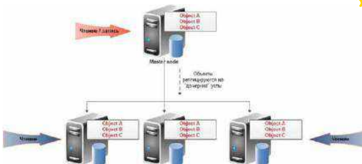
Рис. 22. Master-slave
