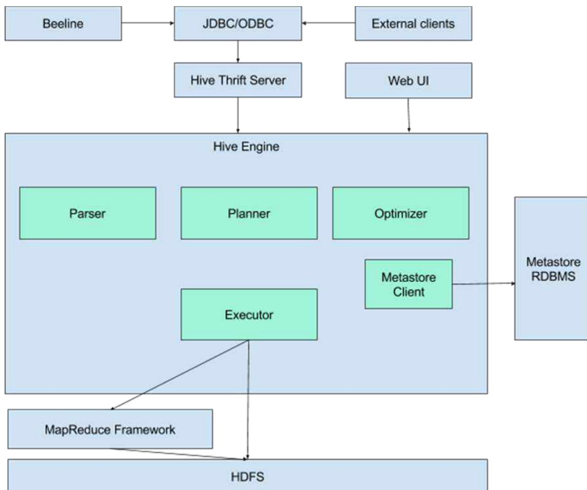
Рис. 27. Архитектура Hive [1]
