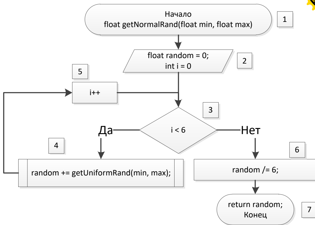
Рис. 6 «Функция getNormalRand»
