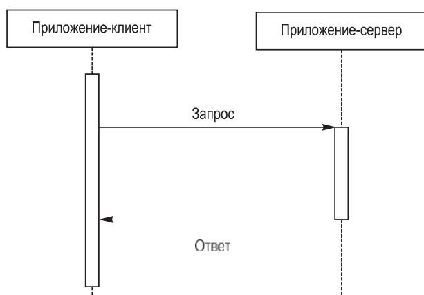
Рис. 2.2. Асинхронное взаимодействие
