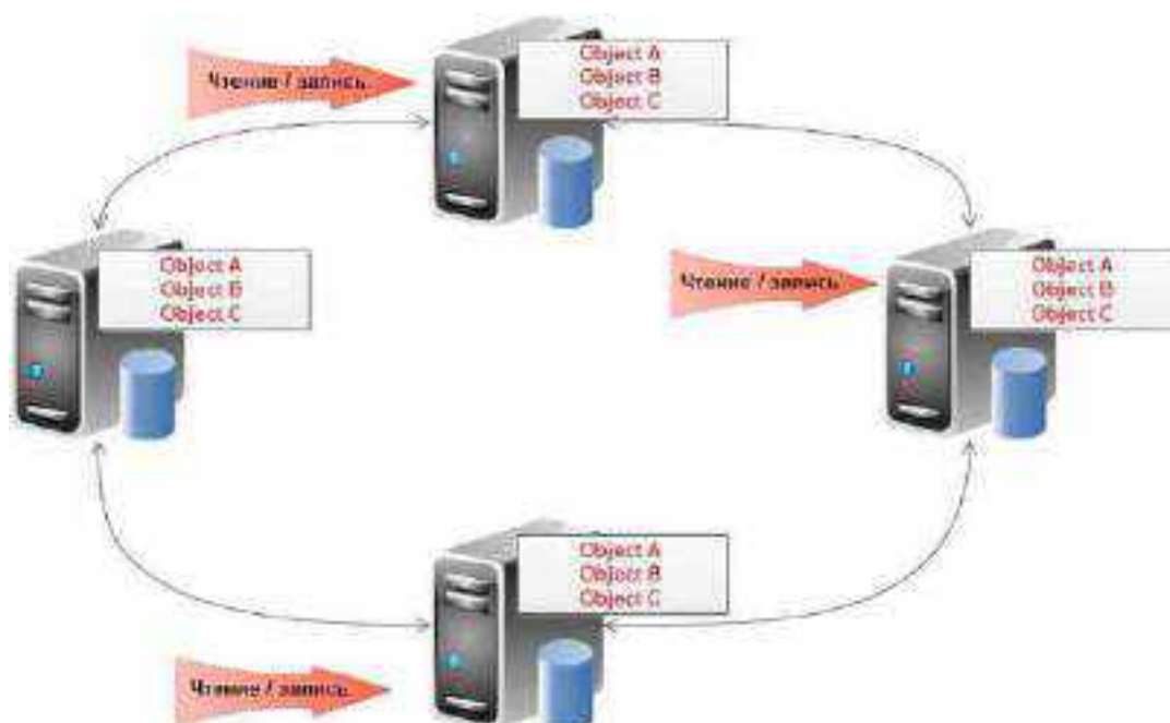
Рис. 23. Peer-to-peer
