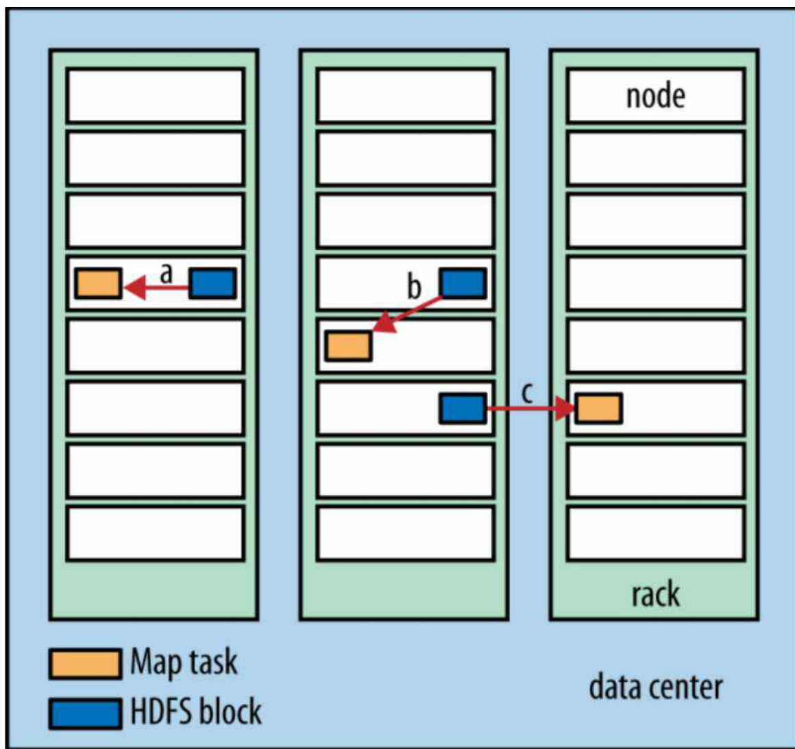
Рис. 12. Возможности split
