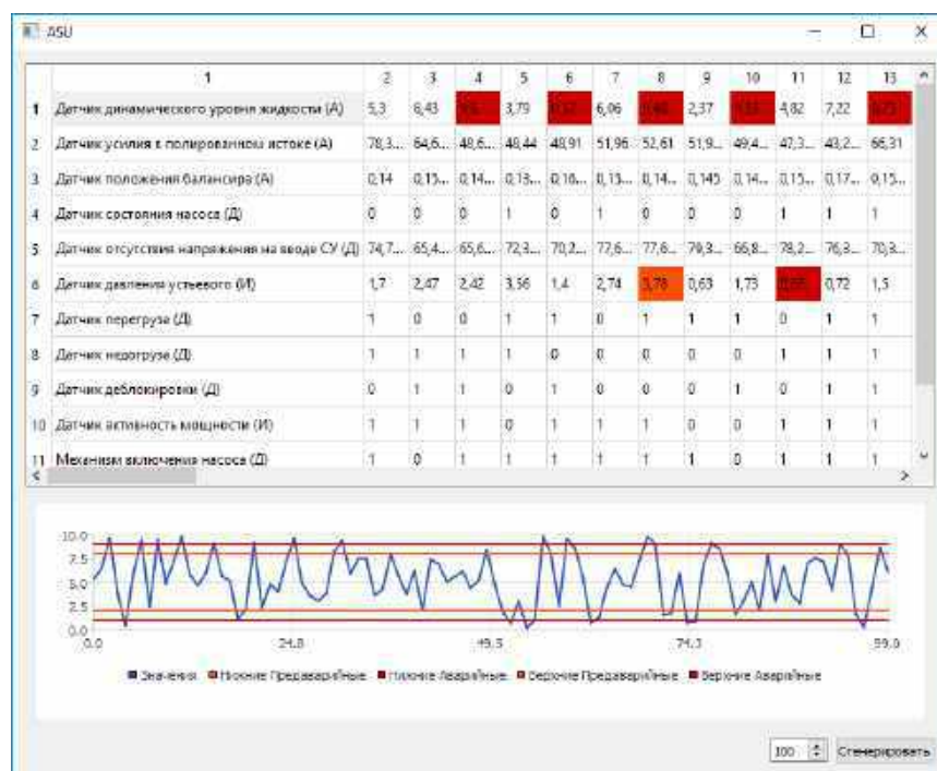
Рис. 10 «Интерфейс программы»
