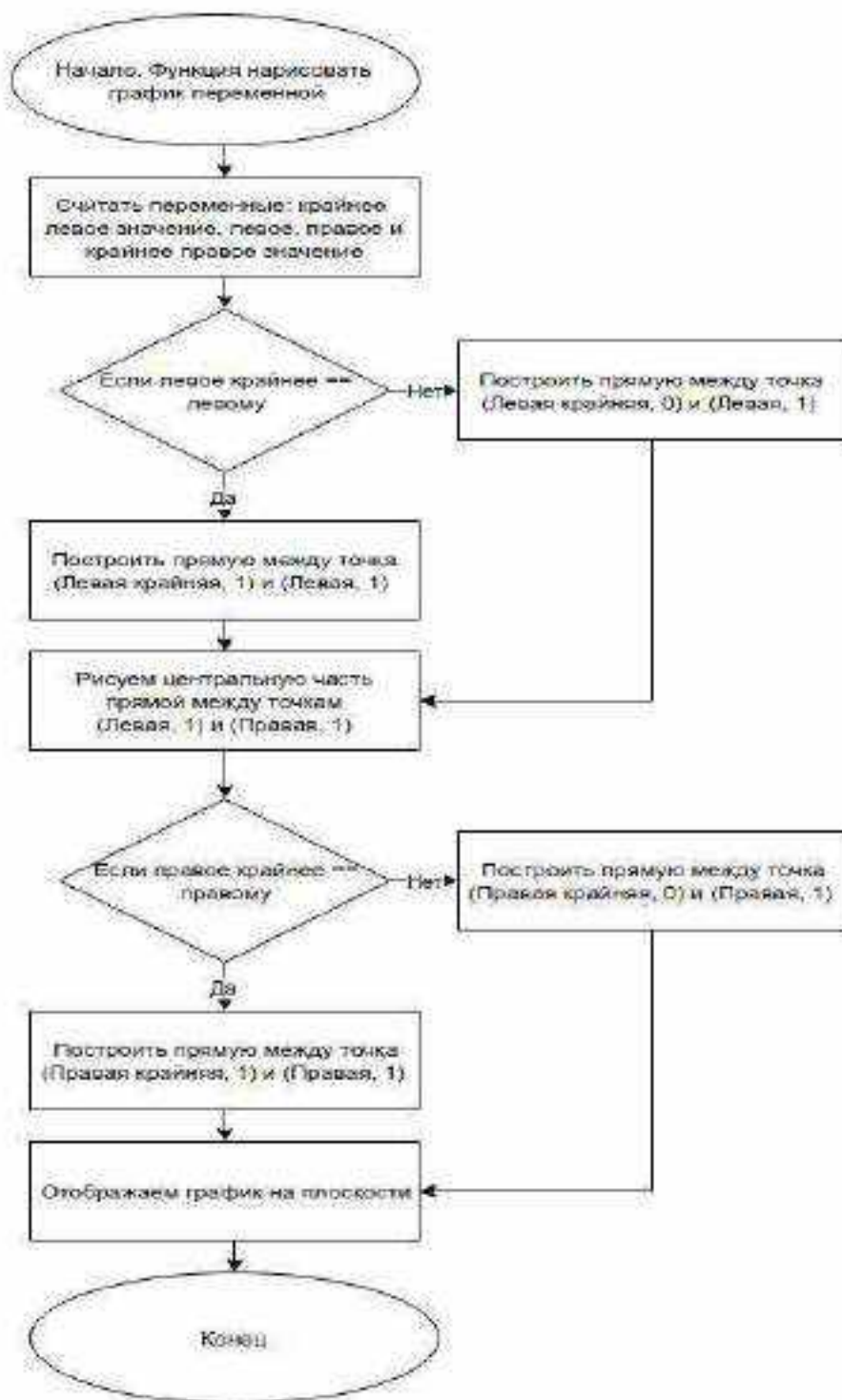
Рис. 18. Алгоритм представления нечеткой термина Алгоритм проверки нечеткой переменной представлен ниже на рисунке 19.
