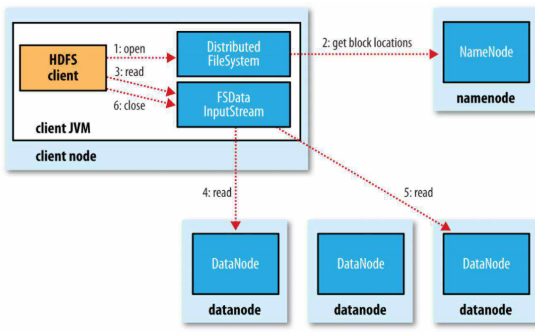
Рис. 17. Основная последовательность событий при чтении файла
