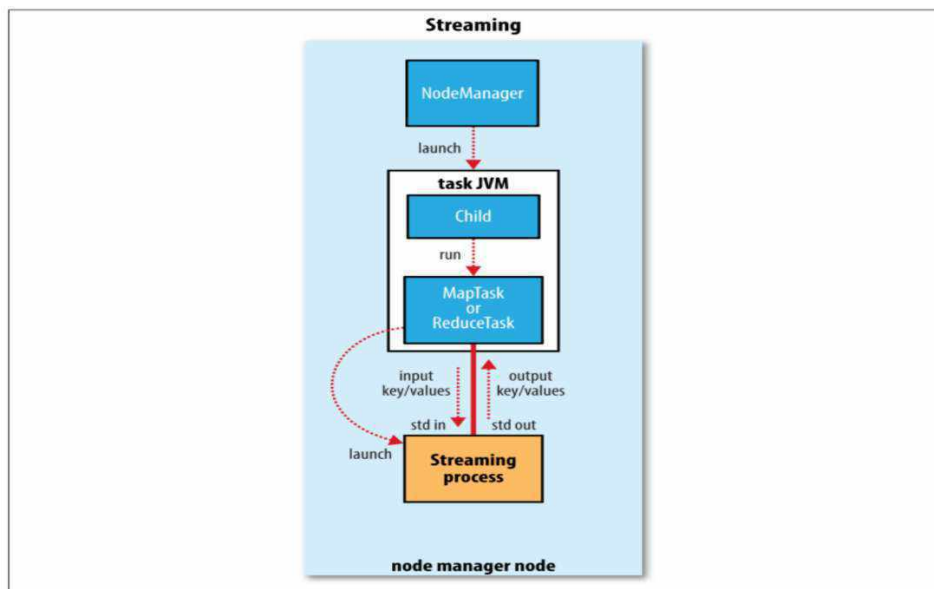
Рис. 34. Поточковая передача данных
