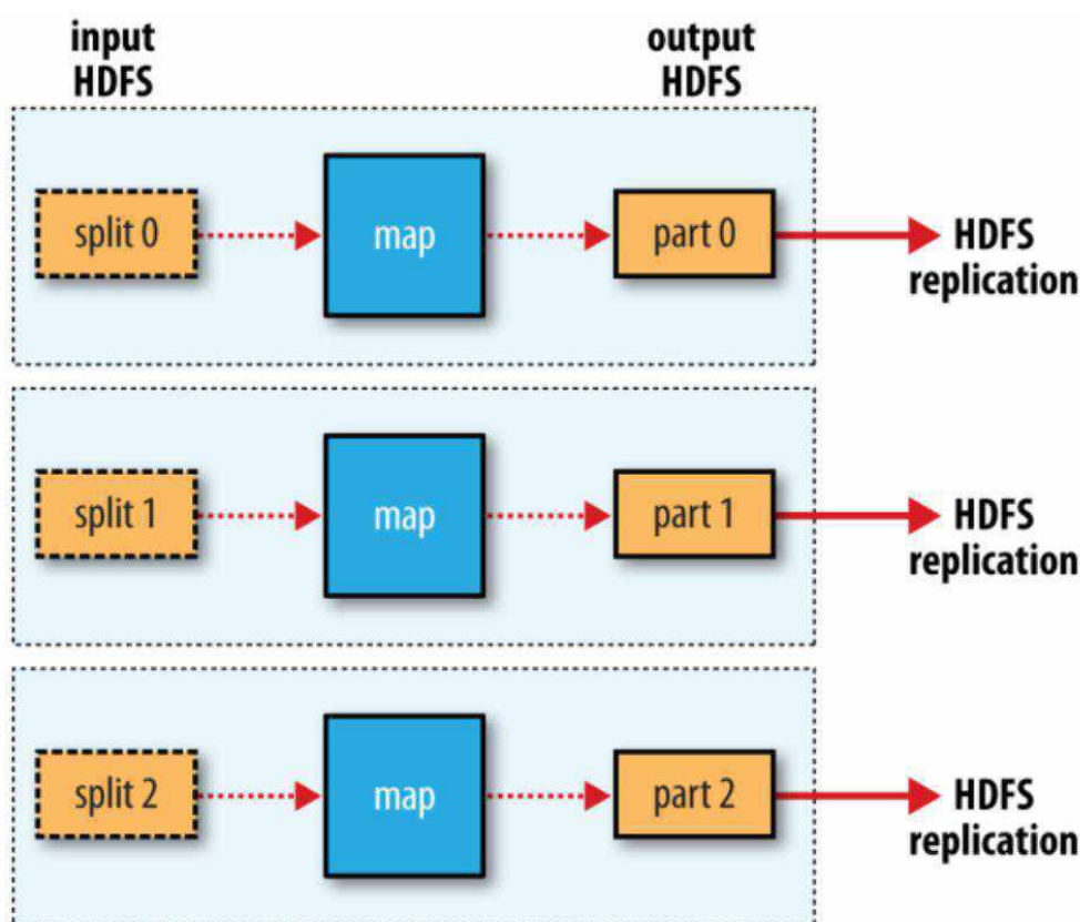
Рис. 15. Параллельная обработка
