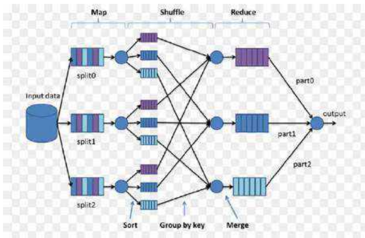
Рис. 11. Парадигма MapReduce
