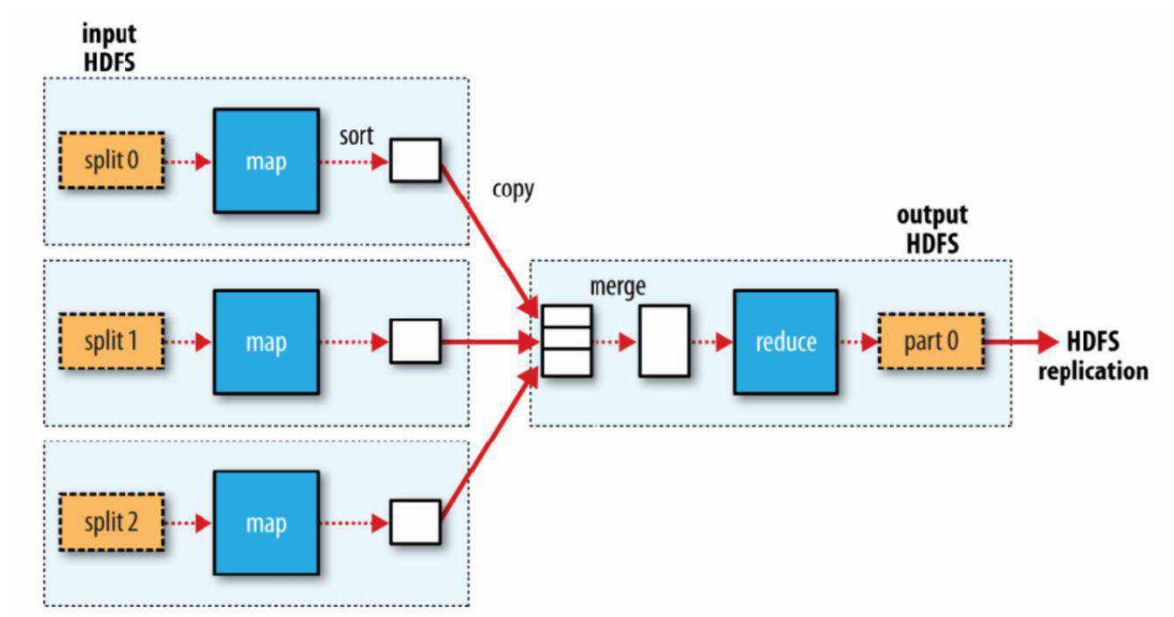
Рис. 13. Свертка
