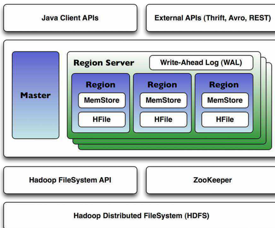
Рис. 26. Архитектура Hbase
