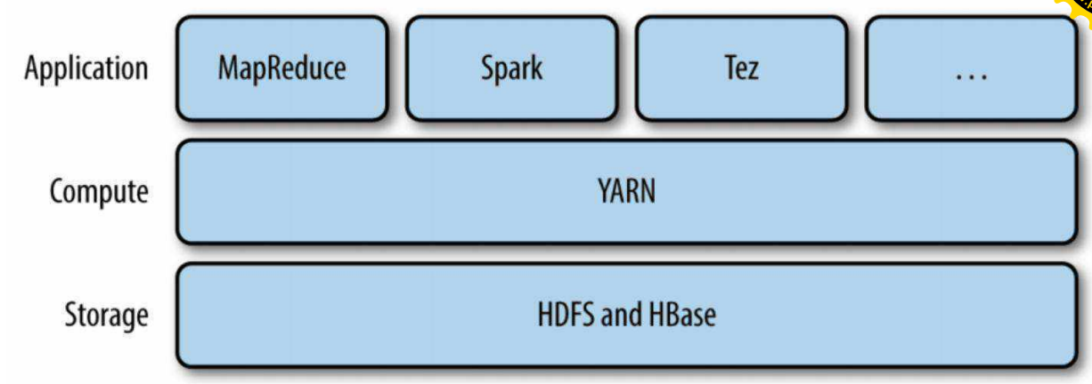
Рис. 31. Многоуровневость YARN
