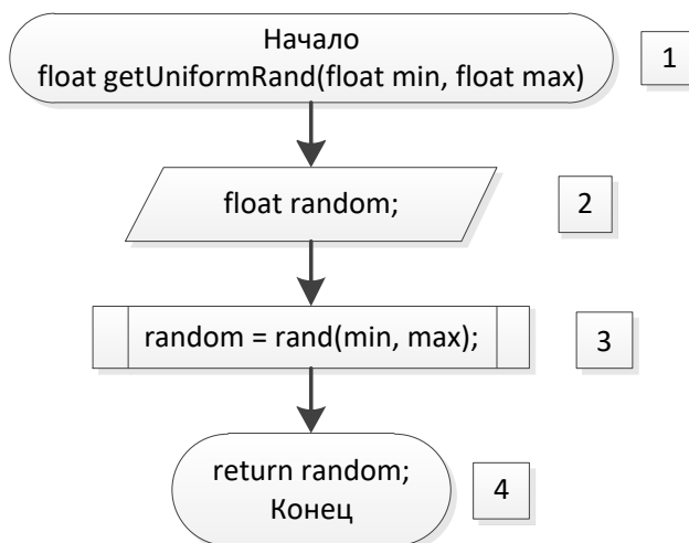
Рис. 5 «Функция getUniformRand»
