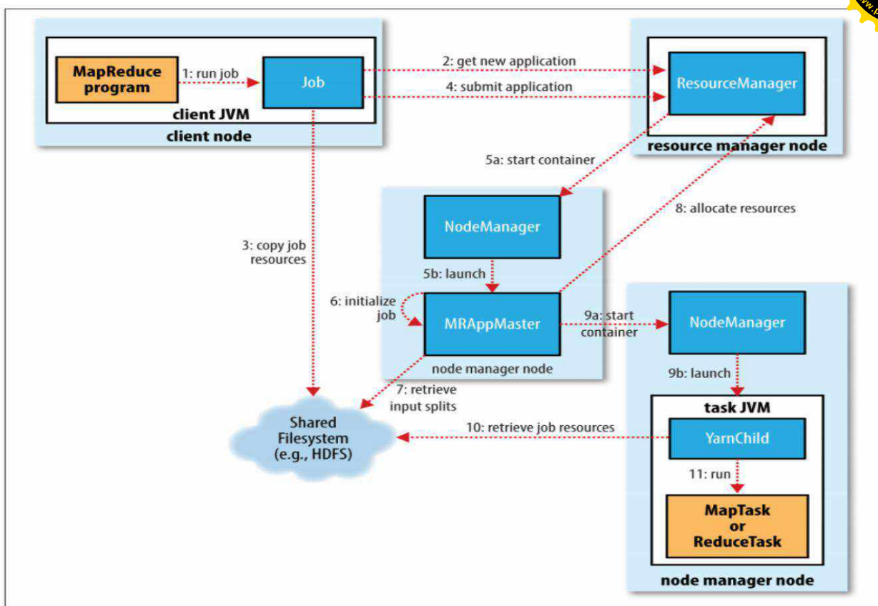
Рис. 33. Процессы MapReduce
