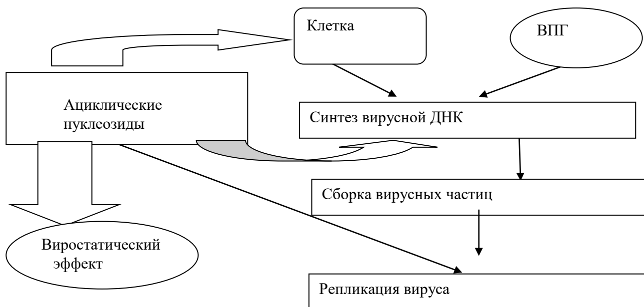
Рис. 1. Механизм действия ациклических нуклеозидов.
