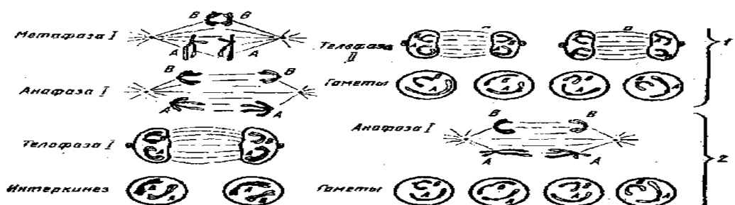
Рис 4. Схема мейоза: 1 и 2 - возможные варианты комбинирования нехомологичных хромосом в образующихся клетках.
