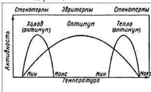
Рис. 1. Эвритермные и стенотермные организмы
