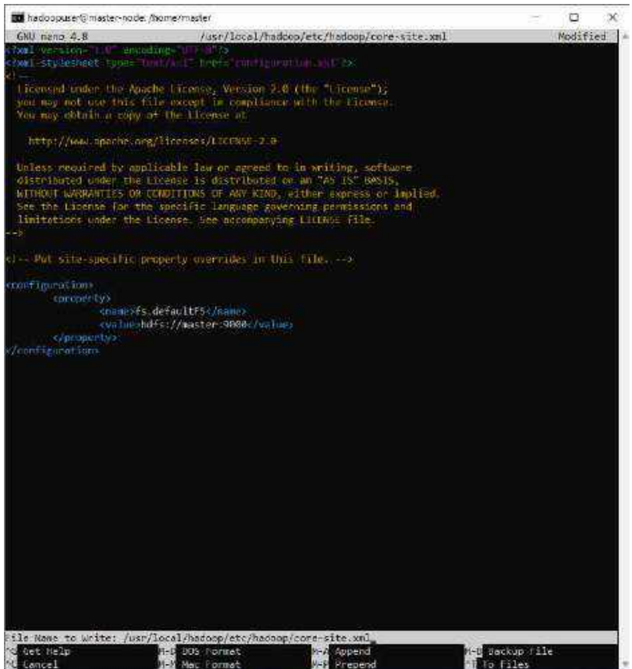
Рис. 30 — процесс настройки портов в конфигурационном файле
