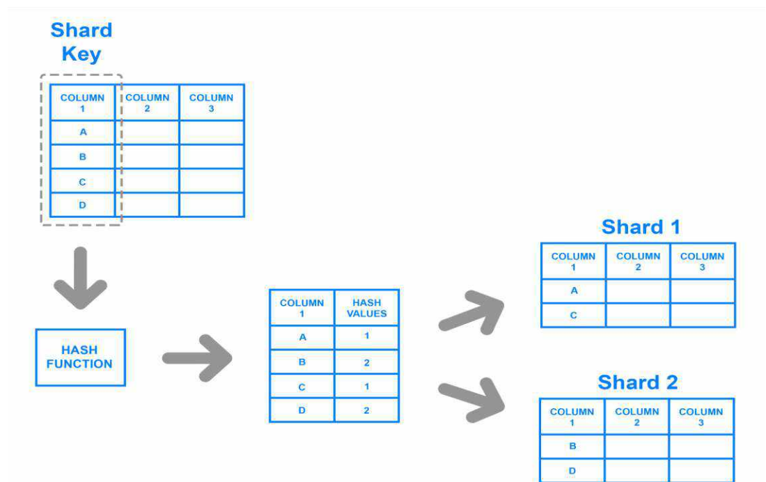
Рисунок 2.2 – Шардинг на основе ключей
