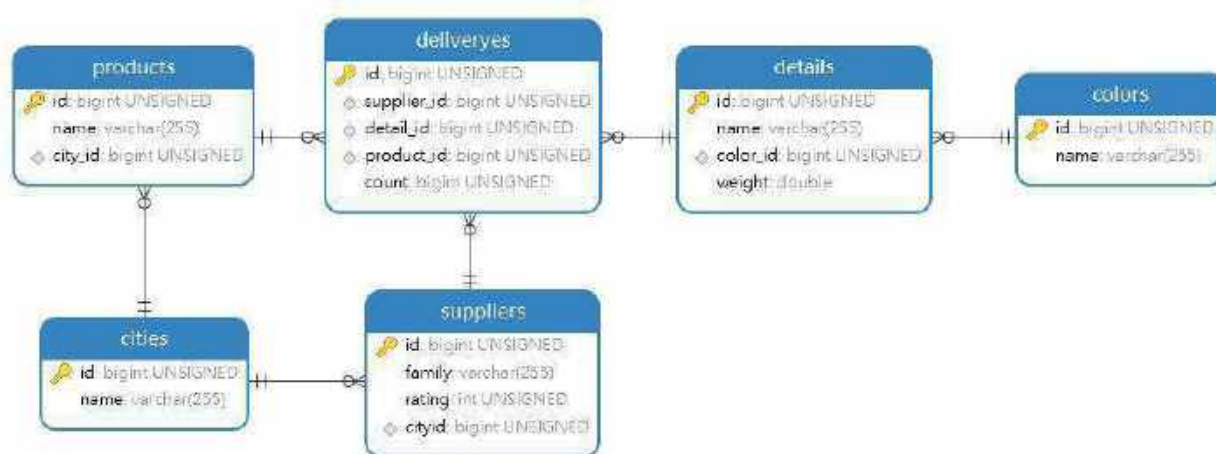
Рис. 17 — Разработанная структура базы данных
