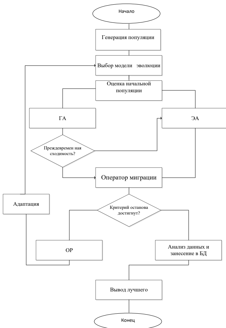
Рис. 2 Обобщенная схема биоинспирированного поиска для задачи об экстремальном пути
