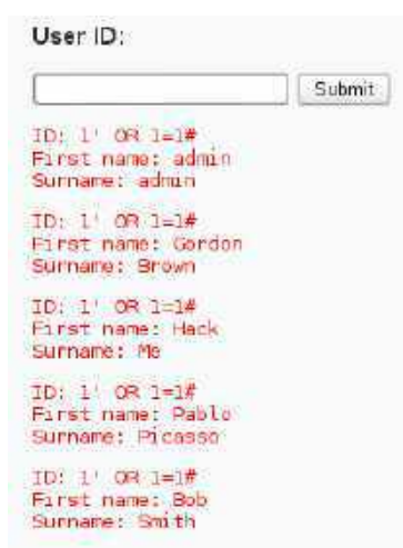
Рис. 1.2. Вывод всех пользователей
