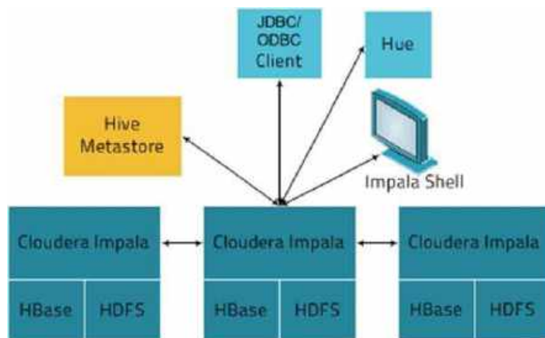
Рис. 28. Архитектура Impala
