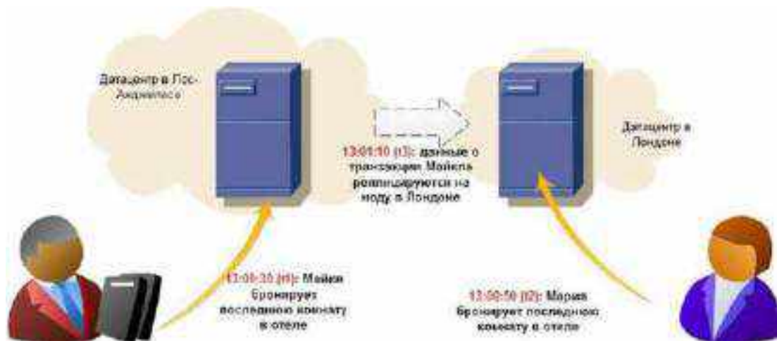
Рис. 21. Рассогласованность данных
