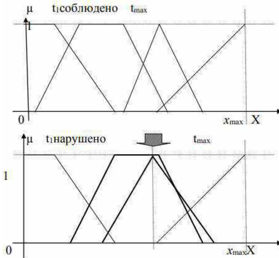
Рис. 16. Разграничение понятий
